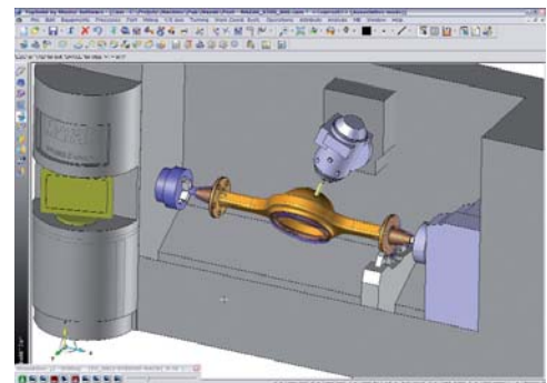
Fräsen mit 4-bzw. 5 positionierten Achsen.
